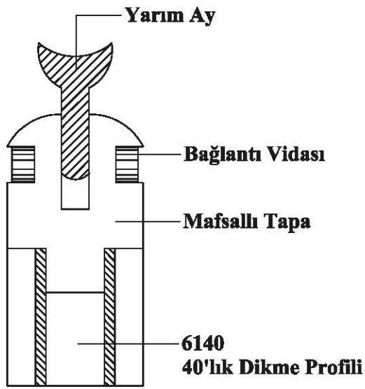
A-A KESİT GÖRÜNÜŞÜ
