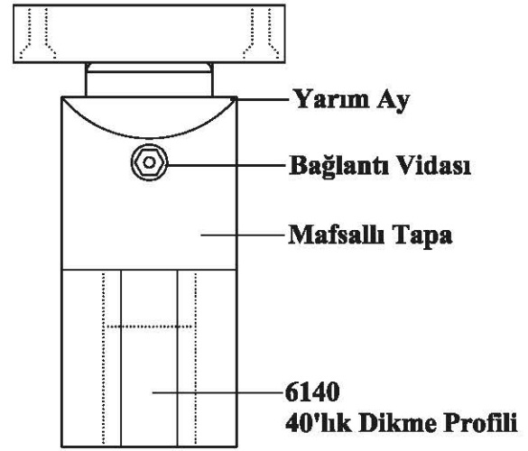
B-B KESİT GÖRÜNÜŞÜ
